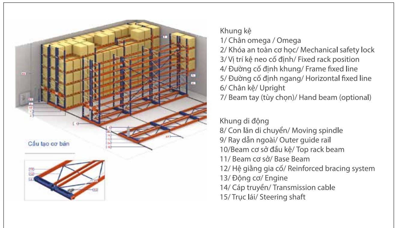
Cấu tạo chi tiết kệ Mobile/ Detail of Mobile Rack
