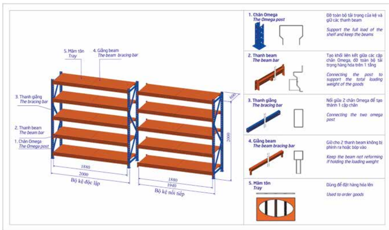
Chi tiết cấu tạo kệ trung tải / Detail of Medium Duty Rack (1)
