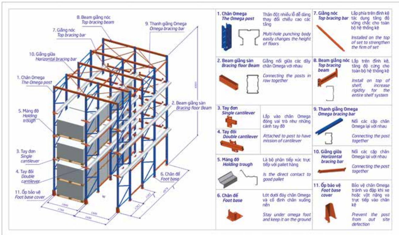
Chi tiết cấu tạo kệ Drive-in/ Detail of Drive-in Rack
