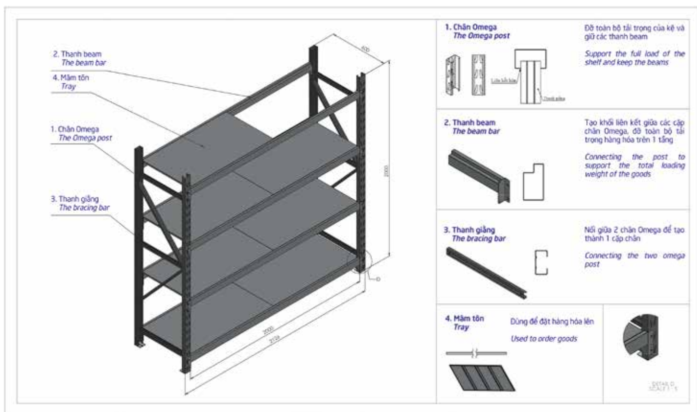
Chi tiết cấu tạo kệ trung tải/ Detail of Medium Duty Rack (3)
