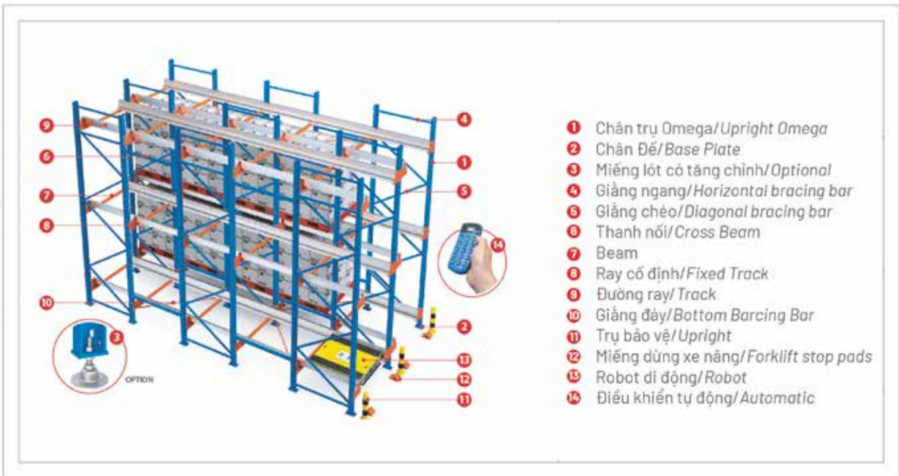
Cấu tạo chi tiết kệ Shuttle/ Detail of Shuttle Rack
