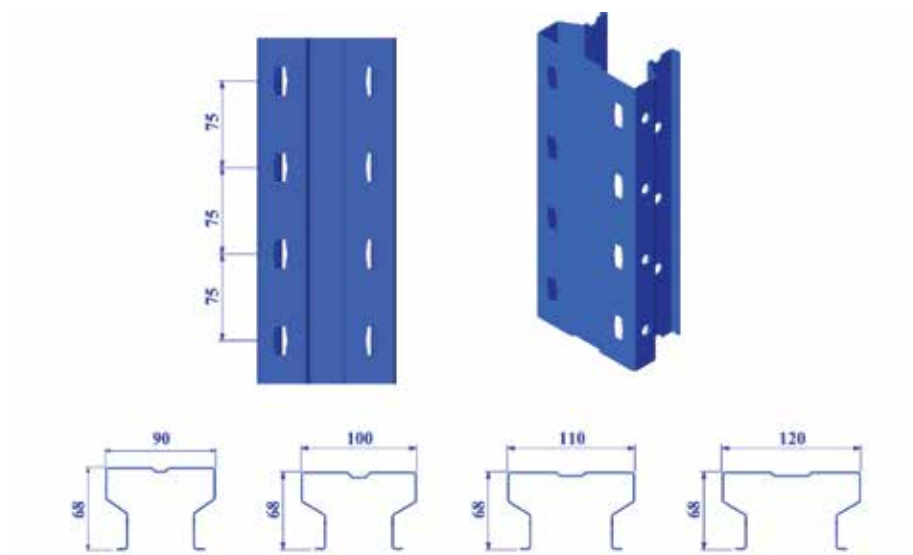
Mặt cắt Omega/ Cross section Omega
