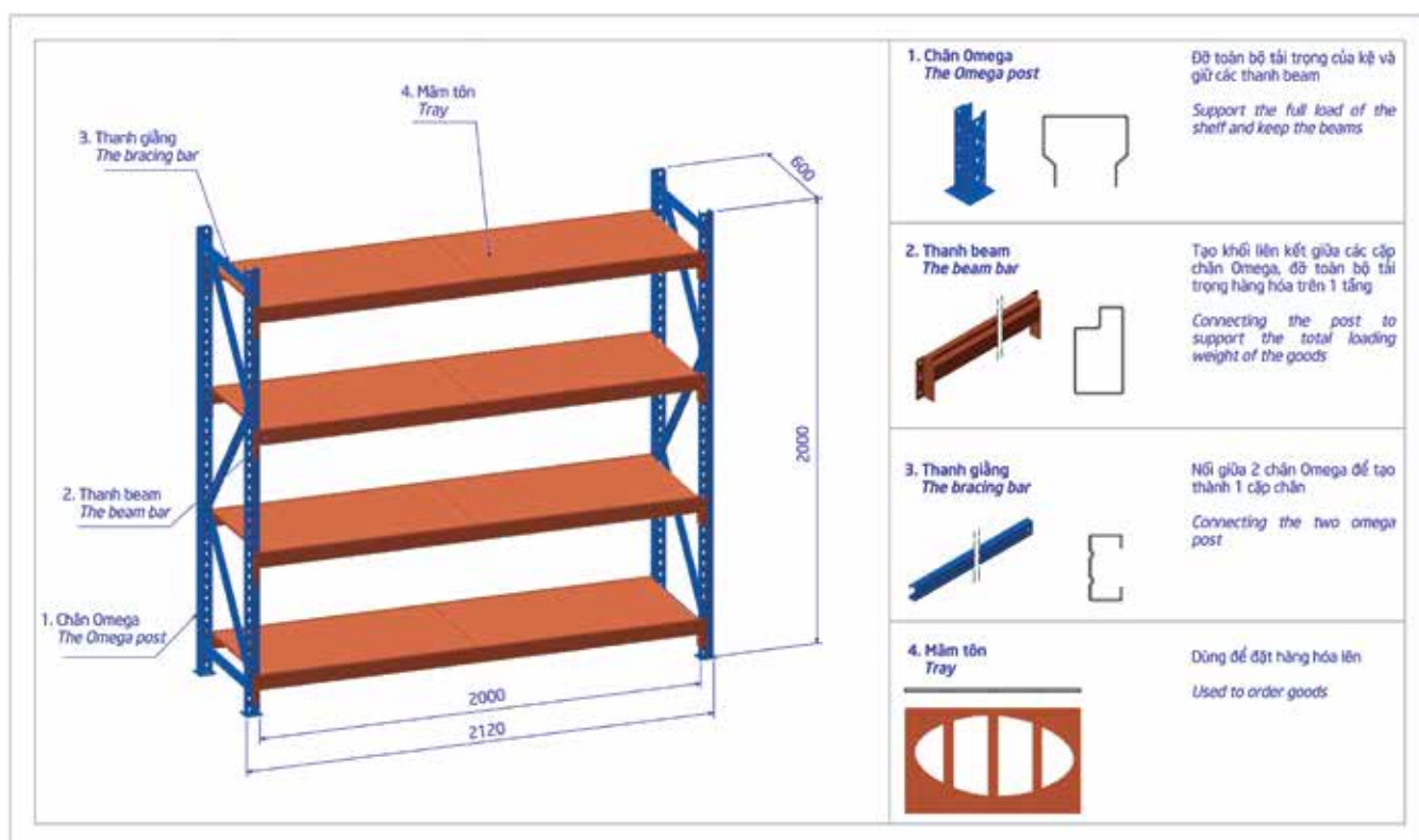
Cấu tạo kệ trung tải/ Detail of medium duty rack
