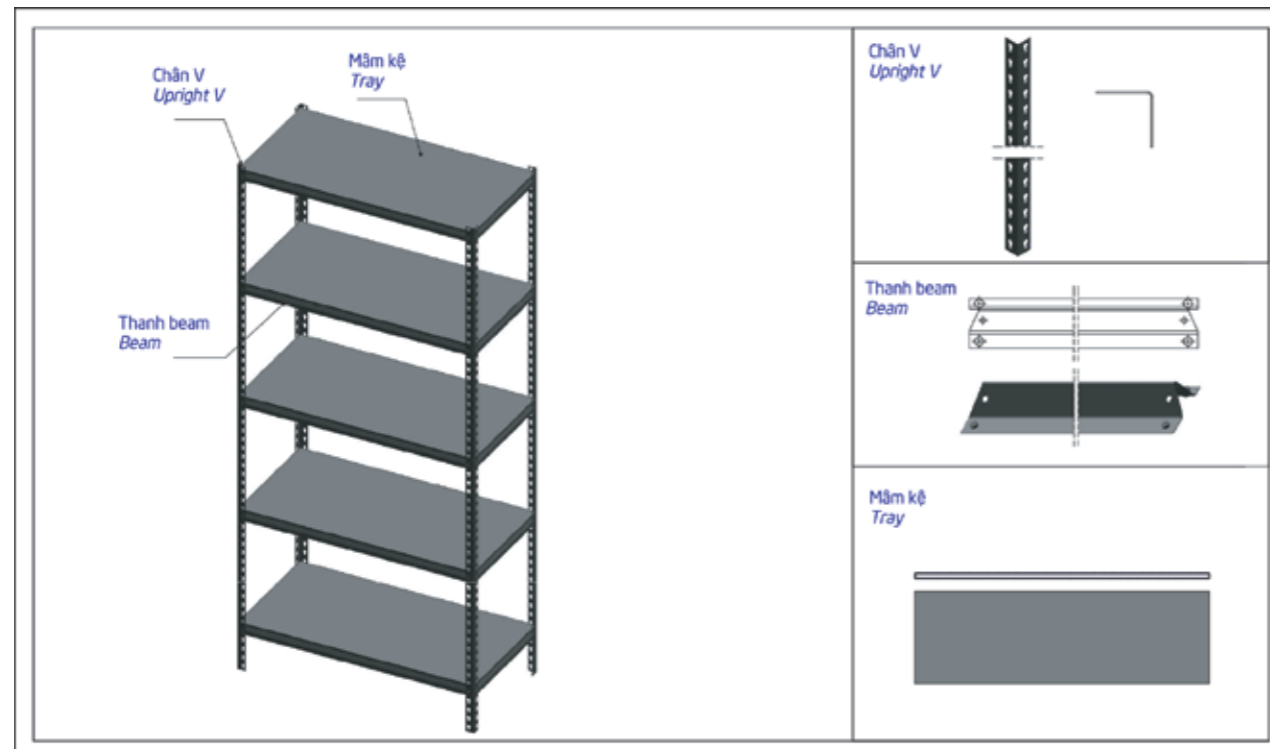
Chi tiết cấu tạo kệ V Vinatech/ Detail of Angel Slotted Rack
