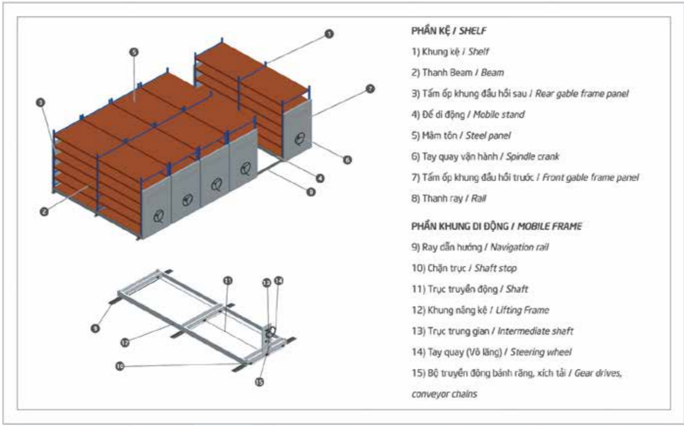
Cấu tạo chi tiết kệ di động tay quay/ Detail of Mobile Shelving
