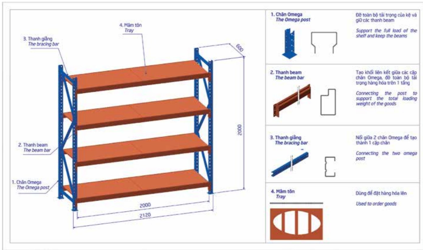
Chi tiết cấu tạo kệ trung tải / Detail of Medium Duty Rack (2)
