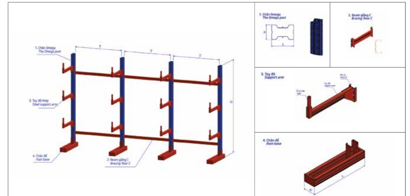
Cấu tạo chi tiết kệ tay đỡ/ Cantilever Rack structure
