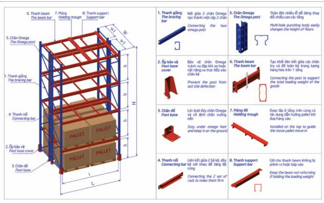
Cấu tạo chi tiết kệ Double Deep/ Detail of Double Deep Rack
