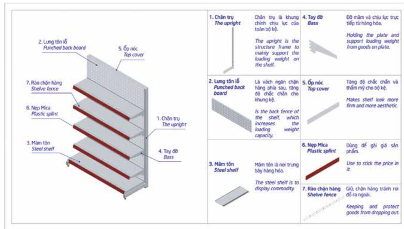
Thiết kế chi tiết kệ siêu thị lưng tôn lỗ / Design of Punched Back Board Type
