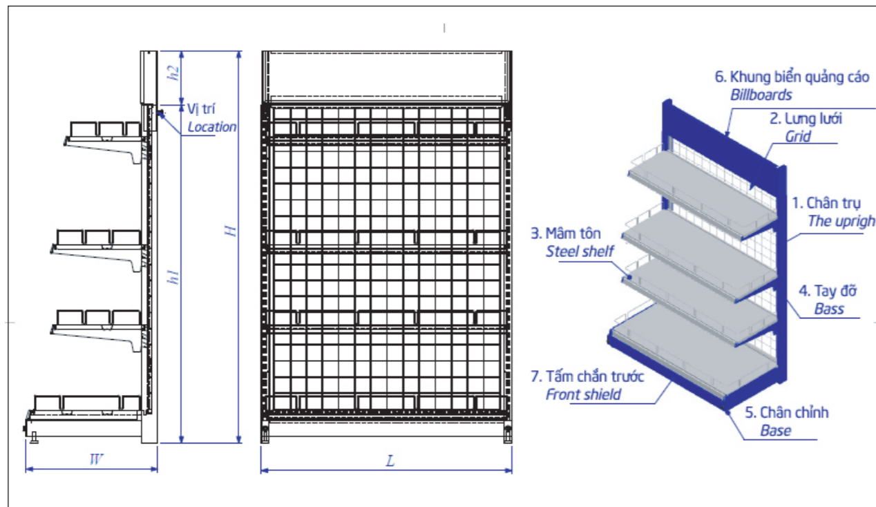
Cấu tạo chi tiết kệ quảng cáo/ Detail of Advertising Shelf
