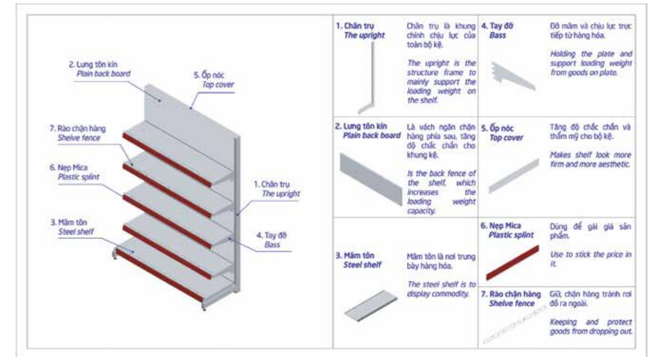
Thiết kế chi tiết kệ siêu thị lưng tôn kín / Design of Plain Back Board Type
